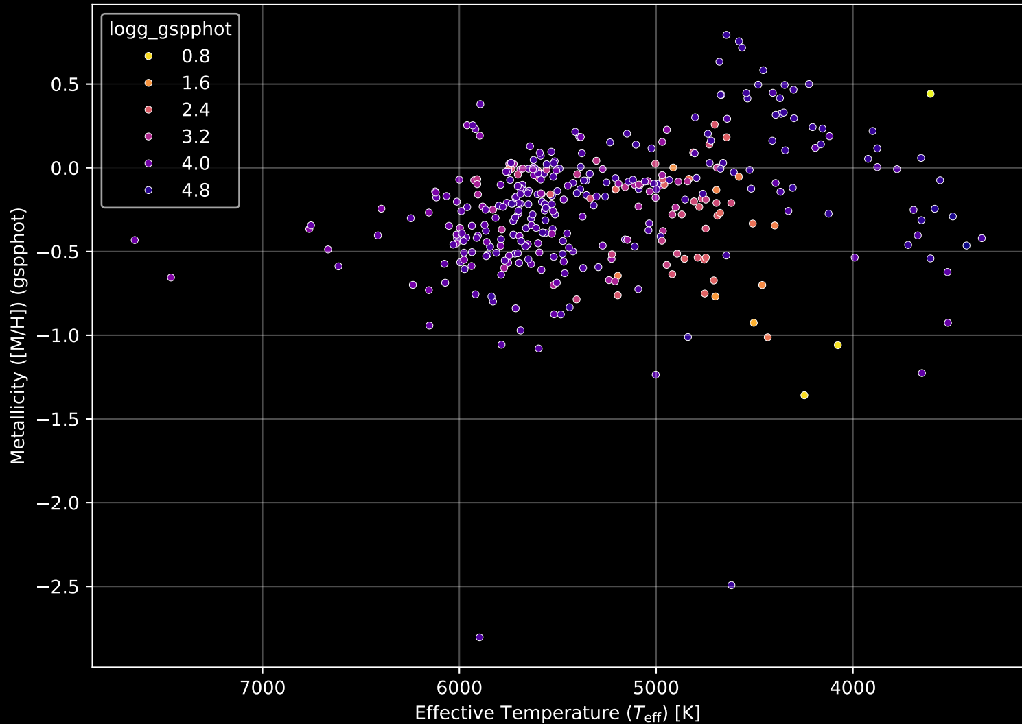
APOGEE DR17 Field: [M79] Stellar Population Parameters (n= 370)
